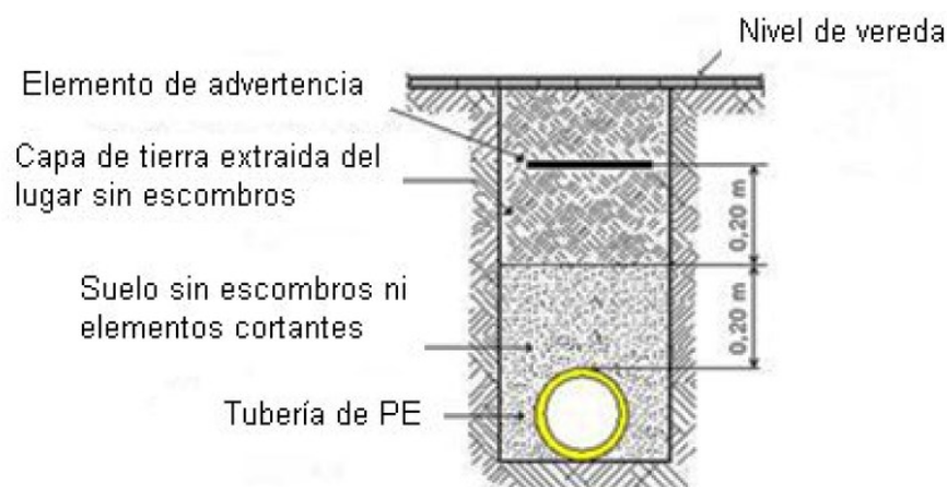
Imagen N° 1.- Tapadas mínimas.
