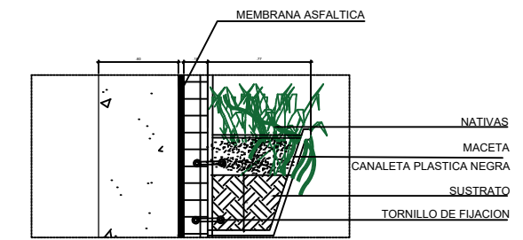
DET. PARED IMPERMEABILIZADA
