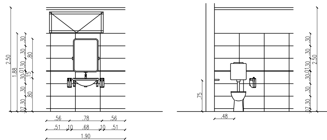
SANITARIOS TIPO SPAZIO ACCESIBLES ESC. 1:50
