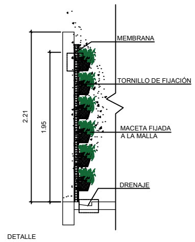
DETALLE
